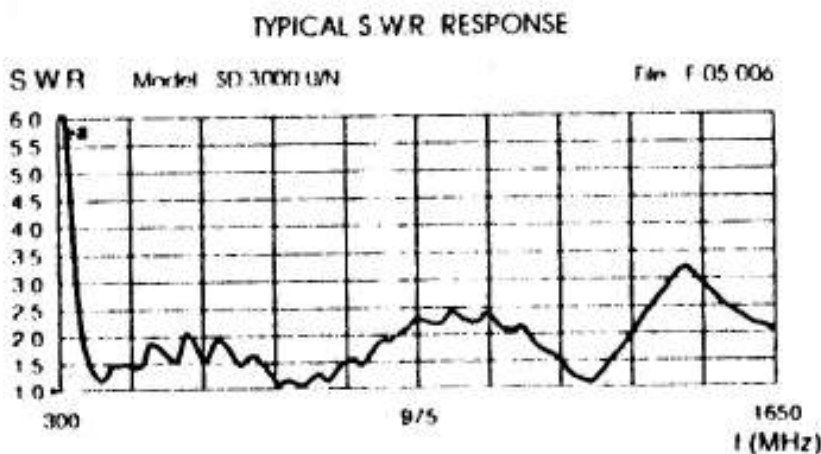
Bild 2: Verlauf des VSWR der Antenne im Frequenzbereich 300 bis 1650 MHz
