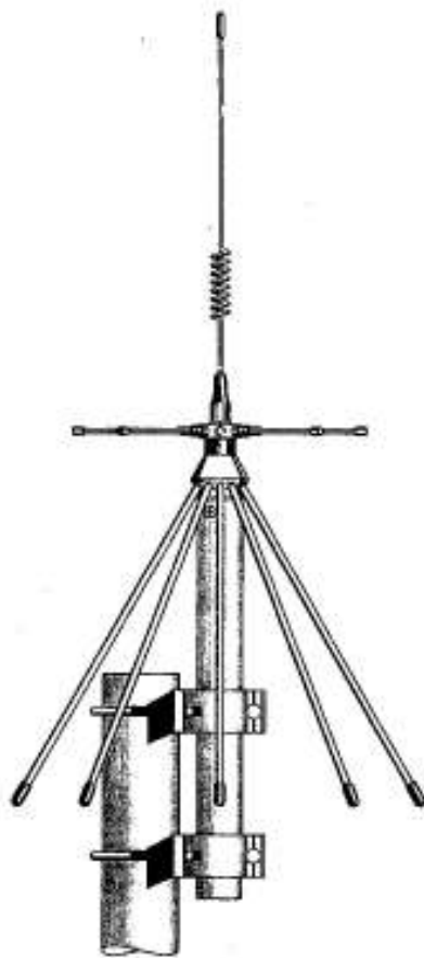
Bild 1: So sieht eine breitbandige Disccone-Antenne aus. Das Antennenkabel wird von unten durch das kurze Rohrstück geführt und an eine N-Buchse angeschlossen
