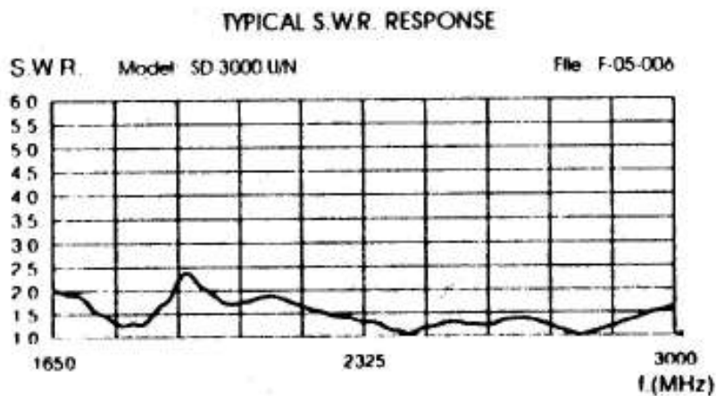
Bild 3: Verlauf des VSWR der Antenne im Frequenzbereich 1650 bis 3000 MHz
